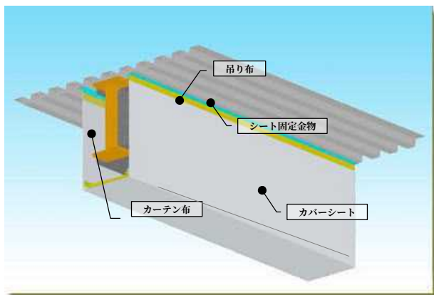
アスベスト密閉時 設置状況
