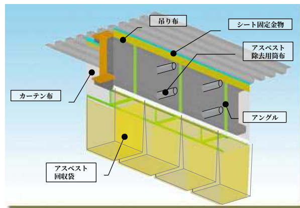
アスベスト除去時 保護シート展開状況
